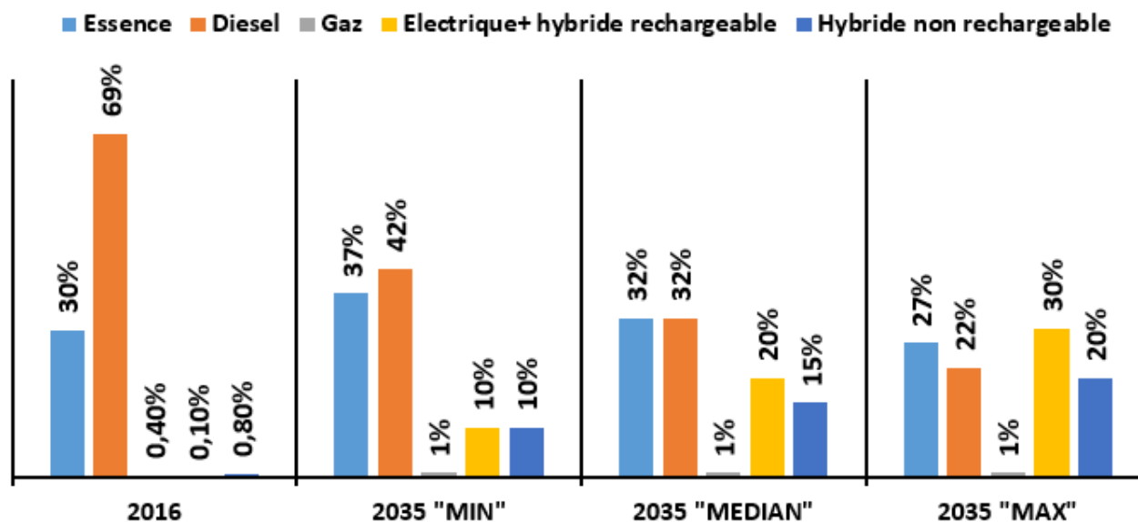
Figure 2. Structure du parc automobile aux différents horizons
