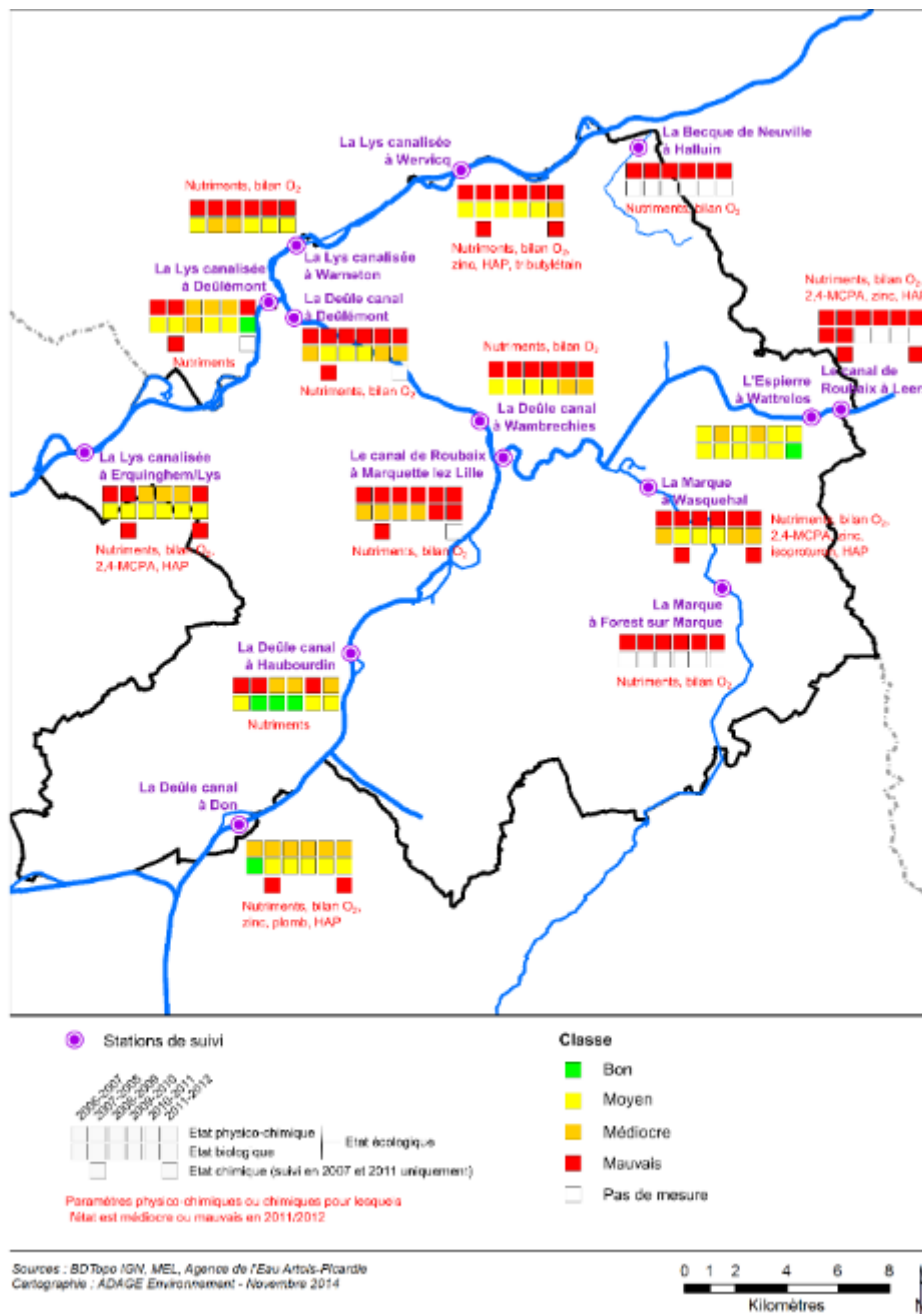
Figure 63. Synthèse de la qualité des cours d'eau de 2006 à 2012
