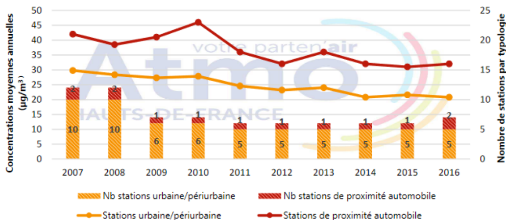
Figure 23. Evolution des concentrations annuelles du NO 2 de la MEL (Source : Stations en activités sur la MEL par année de mesure – Diagnostic de la qualité de l’air ATMO, 2017)
