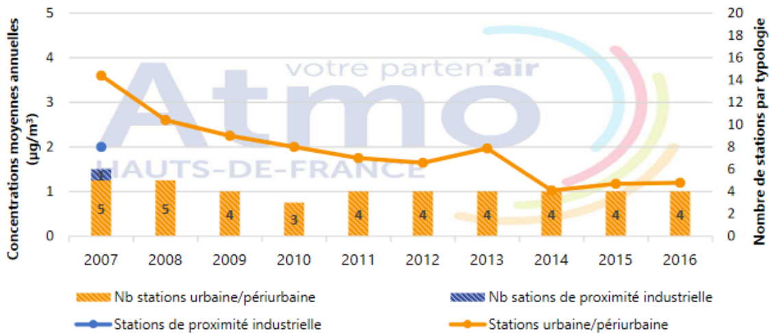
Figure 29. Evolution des concentrations annuelles du SO 2 de la MEL (Source : Stations en activités sur la MEL par année de mesure – Diagnostic de la qualité de l’air ATMO, 2017)
