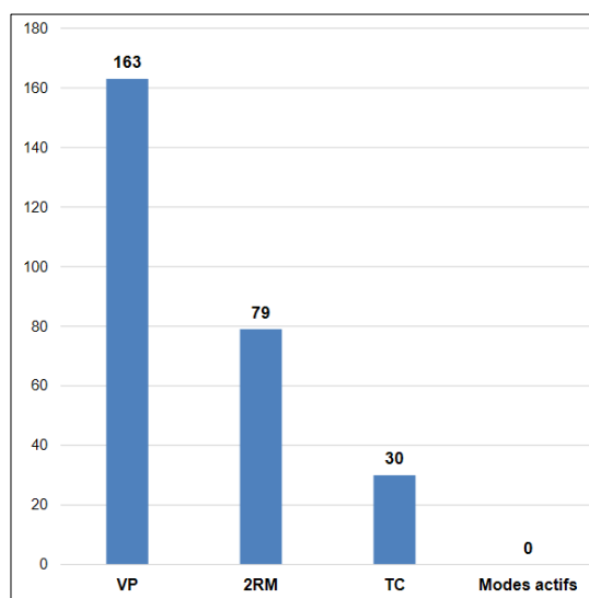
Figure 9. Émissions des GES en g / voyageurs * km (prise en compte uniquement des trajets internes des habitants de la MEL) (Source : Diagnostic Energie Emissions des Mobilités 2016 )
